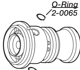
Anode 2083-730ATTC
